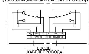
2 x SPST/SPDT Выключатель SRA16, 17, 25 & 40 Для функции 40 контакт NC отсутствует
