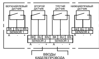
4 x 3-проводной Датчик SRA52 & 53
