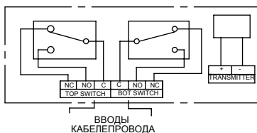
2 x SPST/SPDT и датчик - SRA70 Для SPST контакт NC отсутствует
