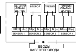
4 x 2-проводной Датчик - SRA52, 53
