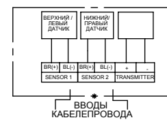
Датчик с 2 x 2-проводной Бесконтактный датчик - SRA70
