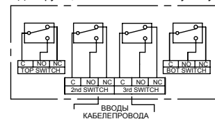
4 x SPST/SPDT Выключатель - SRA55, 56, 58, 59 Для функции 59 контакт N3 отсутствует
