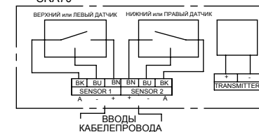
2 x бесконтактный (3-проводной) и Датчик - SRA70
