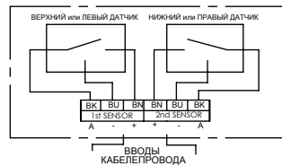
2 x 3-проводной Датчик - SR42, 43
