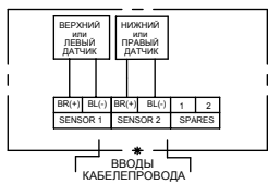
2 x 2-проводной Датчик - SRA42, 43
